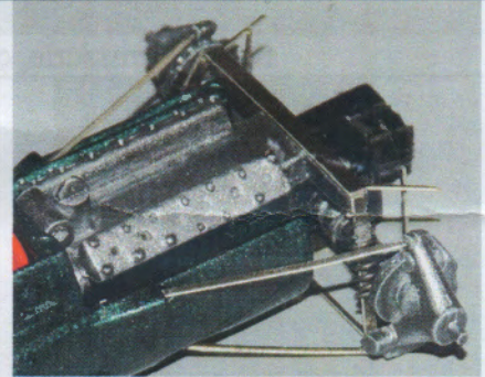
Collez les bras de poussée supérieurs – glue the upper pushrods
