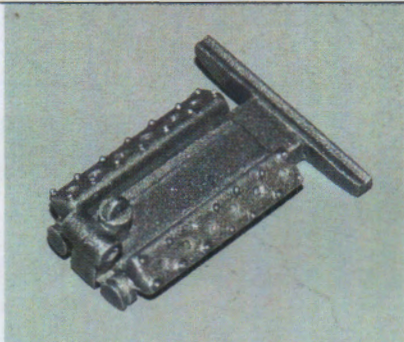
Sur le moteur, collez la partie supérieure de la suspension arrière on the engine, glue the upper part of the rear suspension
