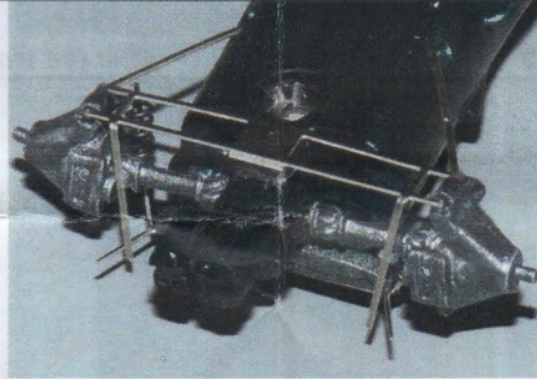
Collez-la ainsi que la transmission et pliez les éléments verticaux – glue it, the transmission to, and fold the vertical parts
